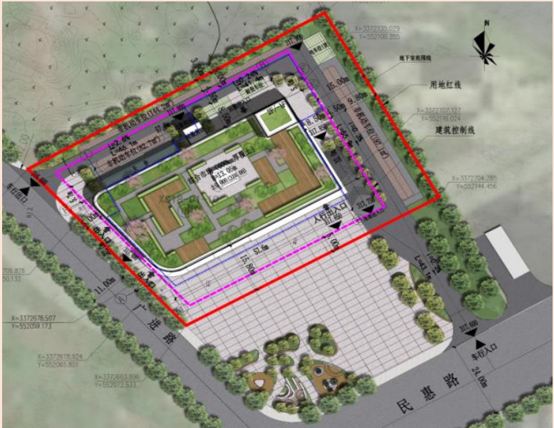
项目总平面图
