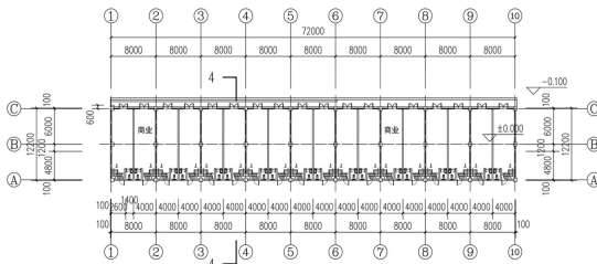
10#楼配套商业1层平面图 1:100
