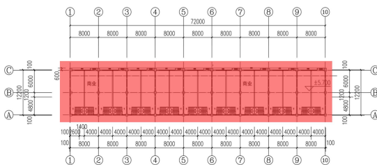
10#楼配套商业2层平面图 1:100
